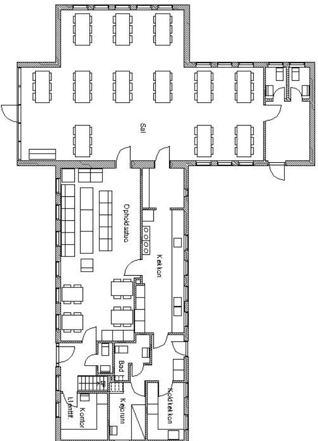
Limbjerggård hovedbygning - plan stueetage
