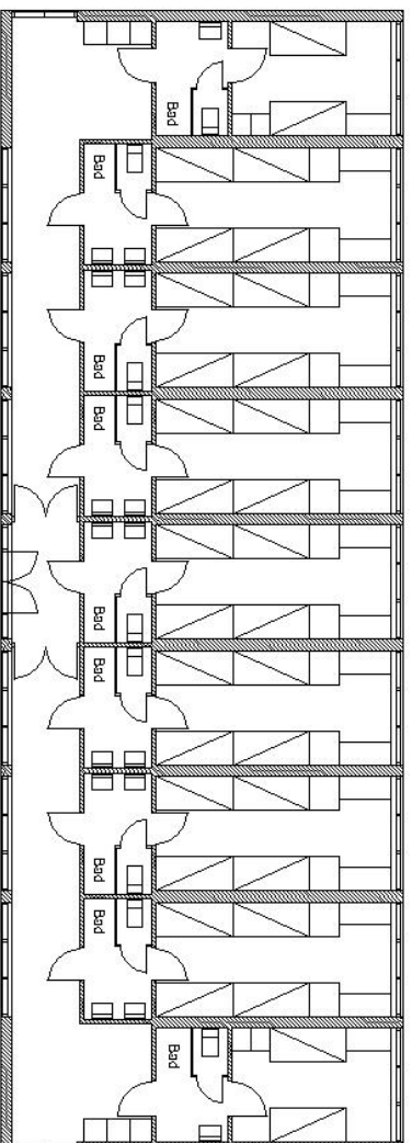
Limbjerggård - plan soverumsbygning
